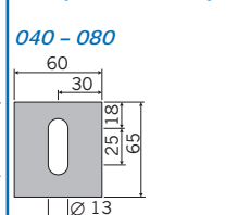
Fußplatte Крепежные элементы для крепления к полу
