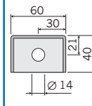
Deckenaufhänger Крепежные элементы для крепления к потолку Ваggröße / Типоразмер 040 - 050 071 - 080
