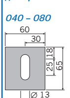
Fußplatte Крепежные элементы для крепления к полу
