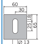
Fußplatte Крепежные элементы для крепления к полу
